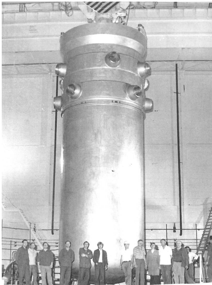
Montáž tlakovej nádoby reaktora V1
