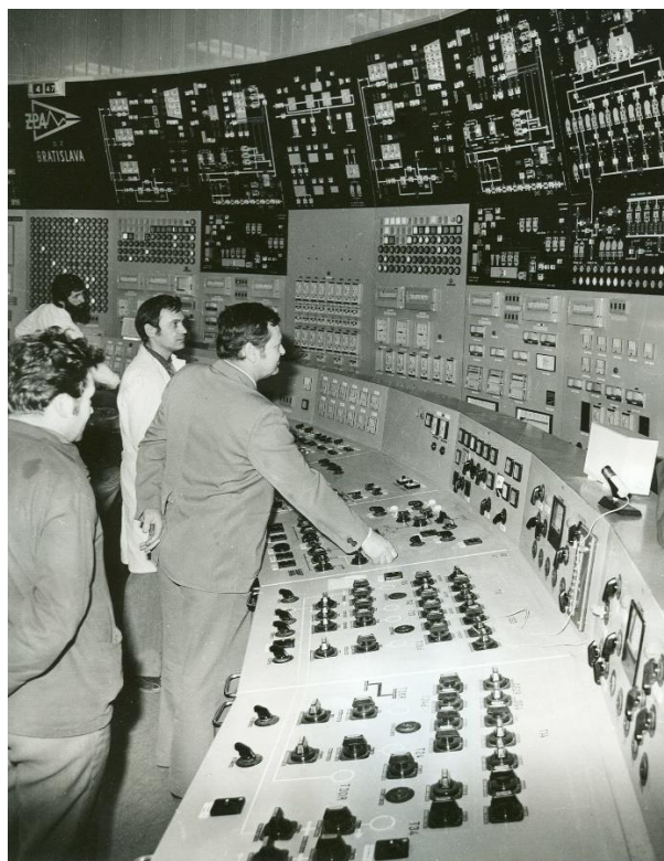
Prvé prifázovanie 2. bloku V1, 1980
