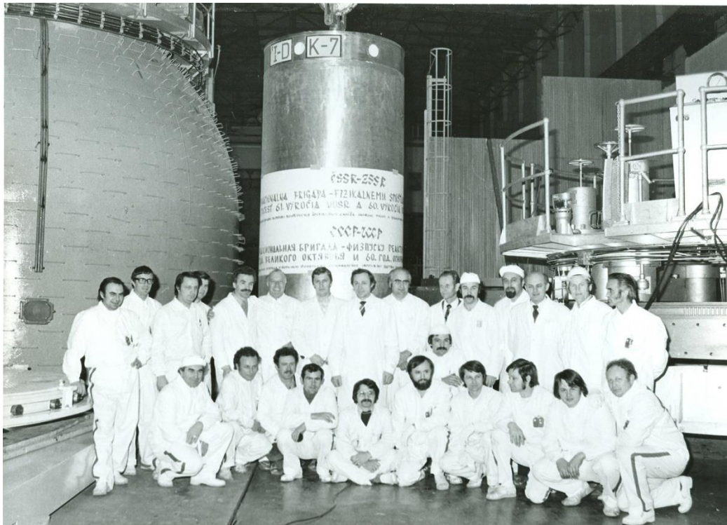
Prvé zavezenie paliva na V1 je pripravené
